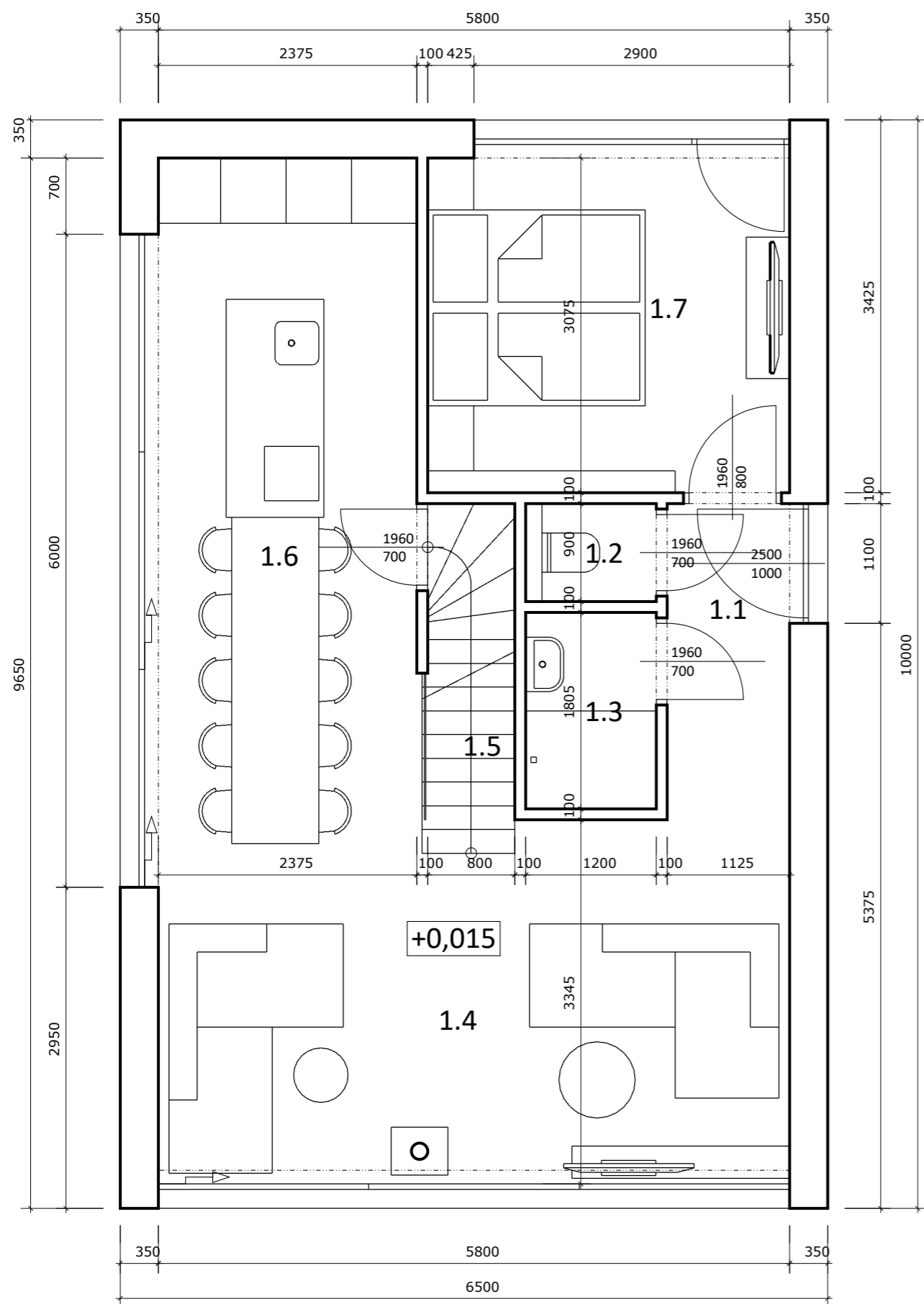
Pôdorys - I.NP, navrhovaný stav, m1:50
