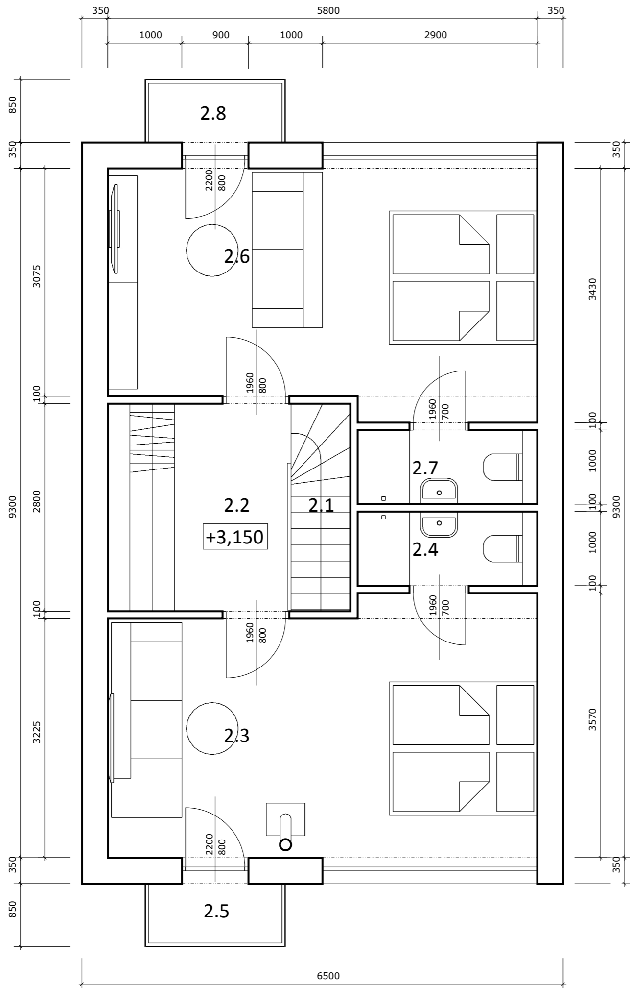
Pôdorys - II.NP, navrhovaný stav, m1:50
